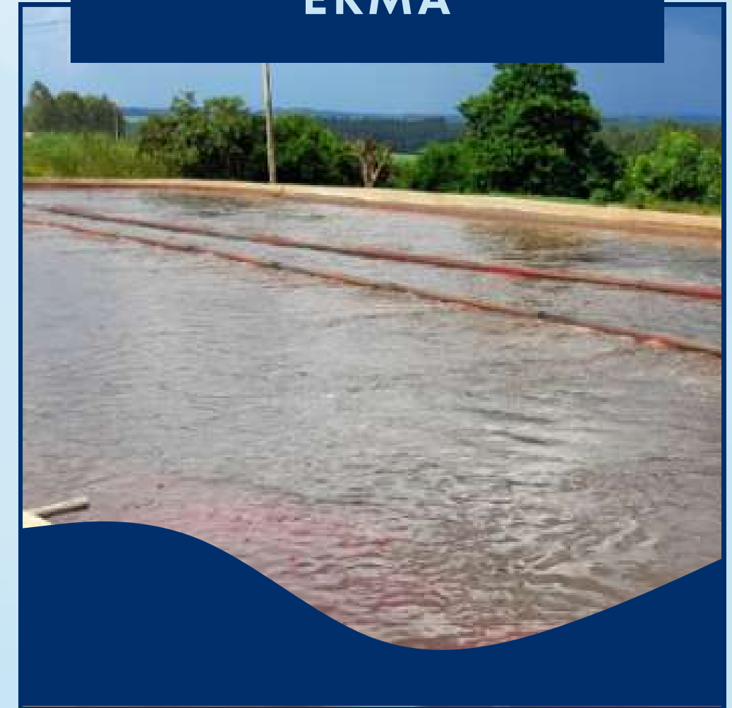
EKMA
